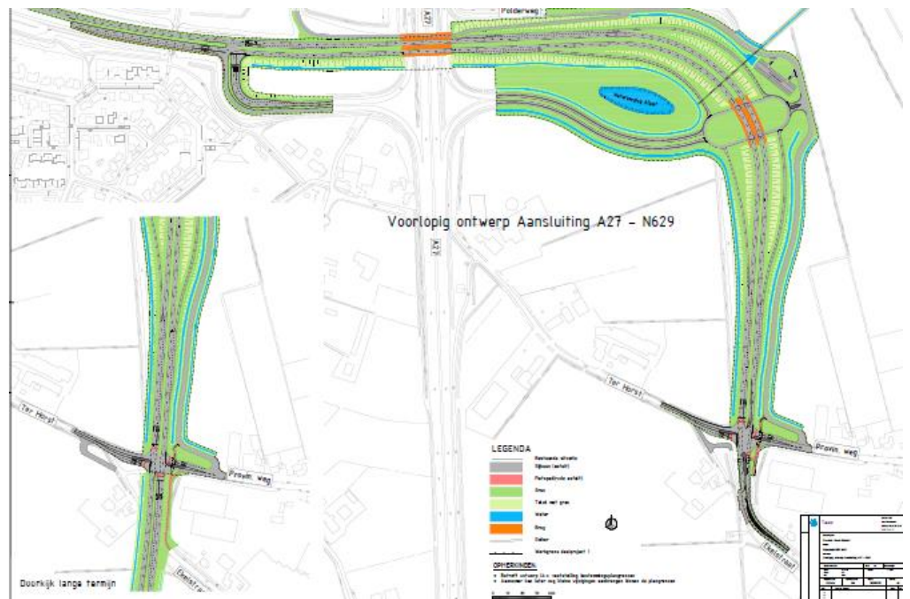
Voorlopig ontwerp aansluiting A27
